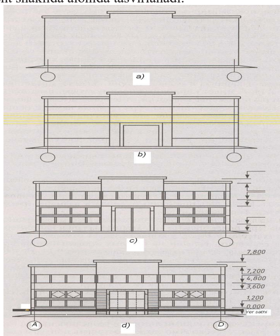
1-shakl. Ishlab chiqarish binosi fasadini chizish bosqichlari
